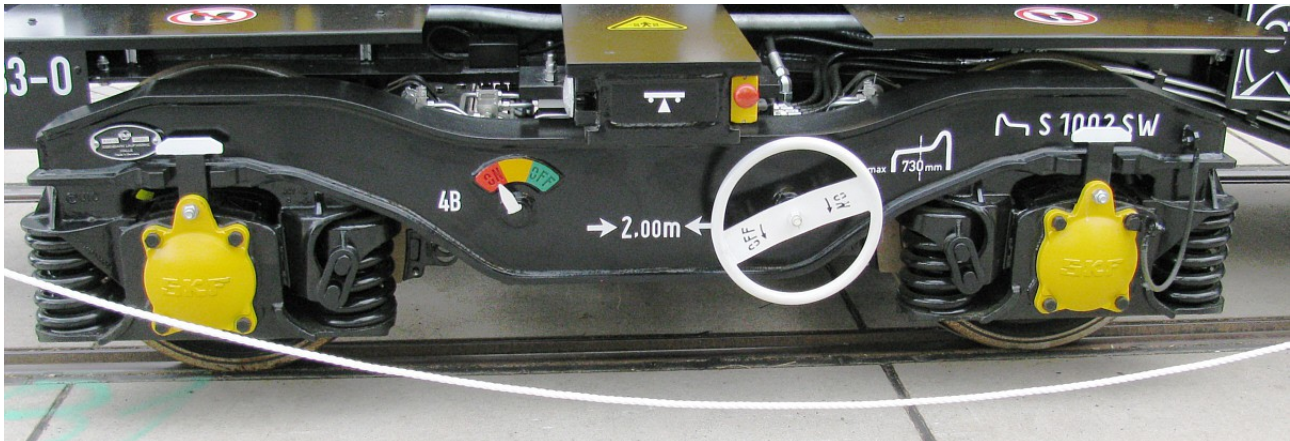
(Dienst-/Maintenance) Güterwagen-Drehgestell//Freight car bogie ELH Y 33 Rsi(f) - UK - block (gesehen auf dem Freigelände unter/seen at the outdoor display with 37 TEN 70 GB -NR 9228 033-0 Uafns/Weichen- Transportwagen)
