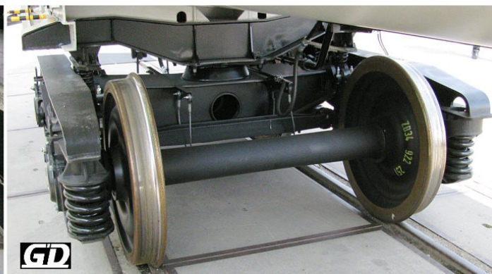
Güterwagen-Drehgestell Astra Y25Lsdi-KC1, gesehen auf dem Freigelände unter 37 TEN 84 NL -GATXD 7818 488-0 Zags Freight Car Bogie Astra Y25Lsdi-KC1, seen at outdoor display with 37 TEN 84 NL -GATXD 7818 488-0 Zags
