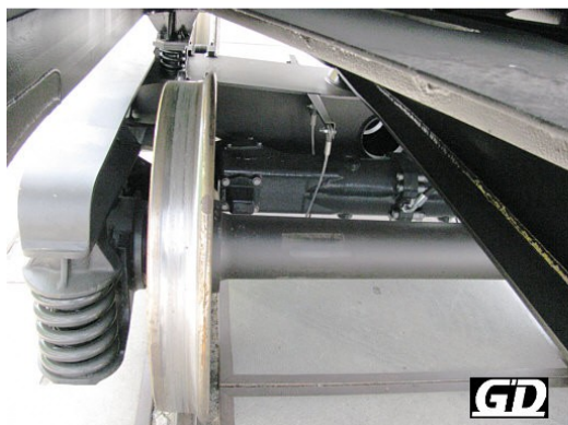
Güterwagen-Drehgestell Astra Y25Lsdi-KC1, gesehen auf dem Freigelände unter 37 TEN 84 NL -GATXD 7818 488-0 Zags Freight Car Bogie Astra Y25Lsdi-KC1, seen at outdoor display with 37 TEN 84 NL -GATXD 7818 488-0 Zags
